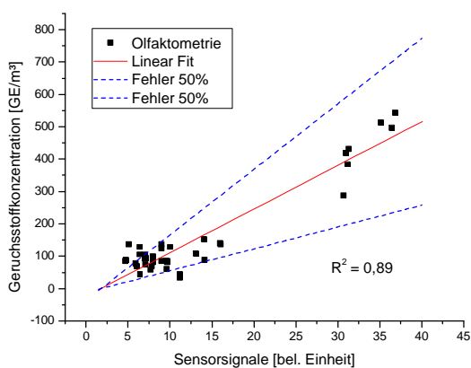
Kalibrationszusammenhang
