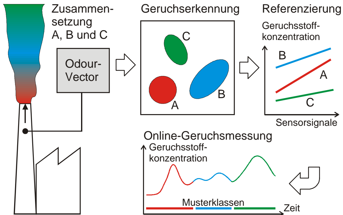
Technisch-sensorische Geruchsmessung mit dem OdourVector™-Meßsystem
